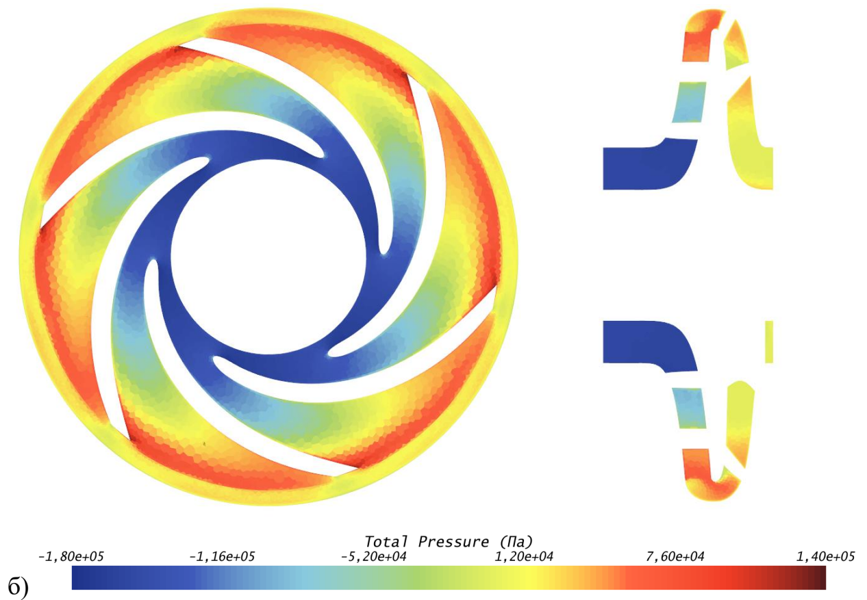
Поля распределения скалярных величин: а) Амплитуды скорости; б) Полного давления.
